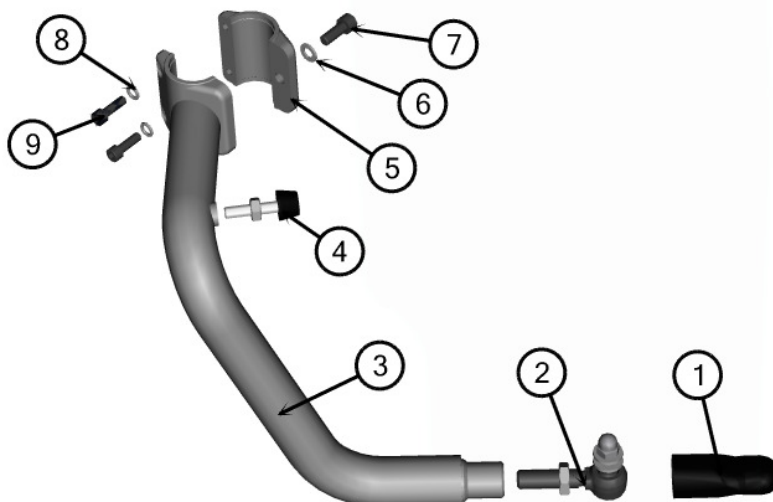
15326.00.D Gr. Braccio Inferiore LOWER ARM ASSEMBLY
